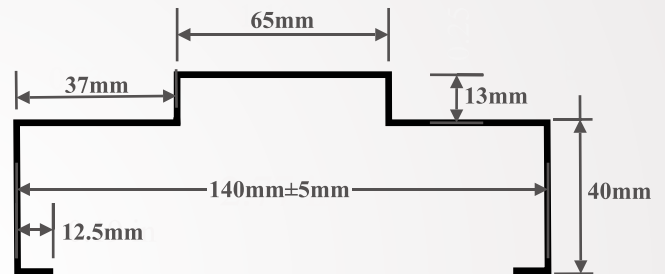
Double Collar Door Frame
